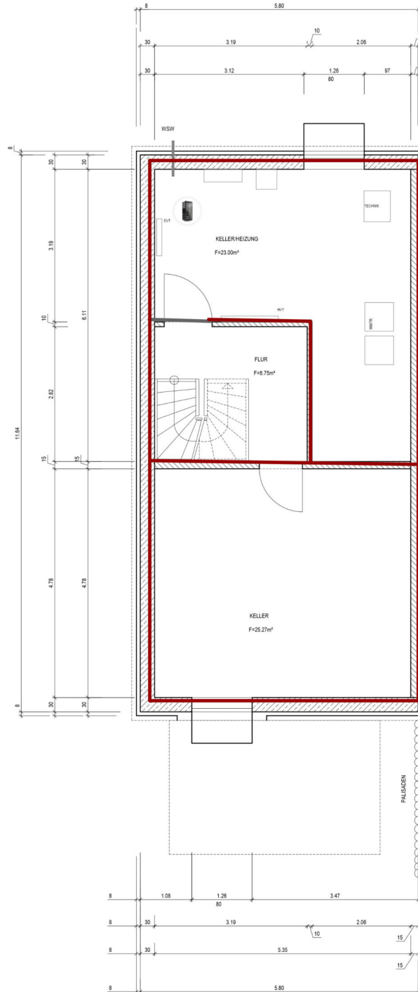
Kellergeschoss M 1:50
